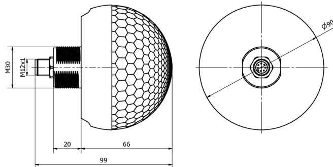
Rozměrový výkres EZ360331
