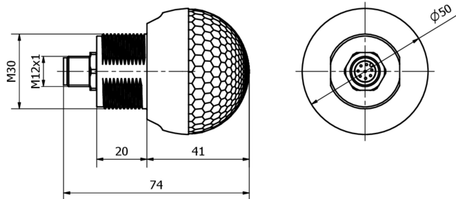
Rozměrový výkres EZ360330
