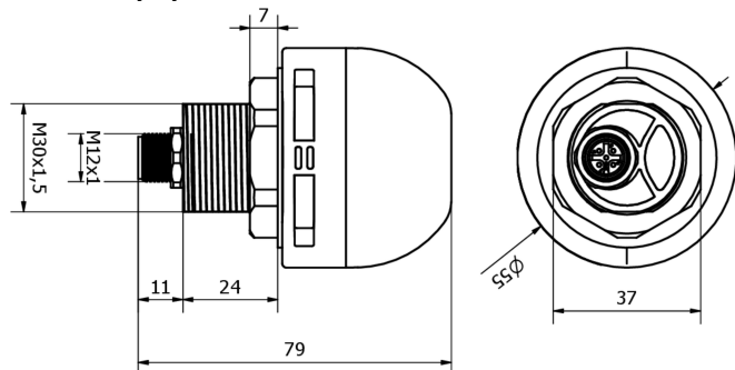
Rozměrový výkres EZ550320
